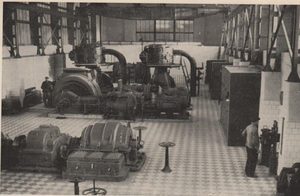
Компресорска станица рудника
