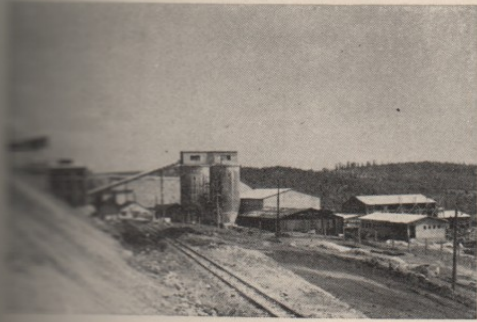
Цијанизација
