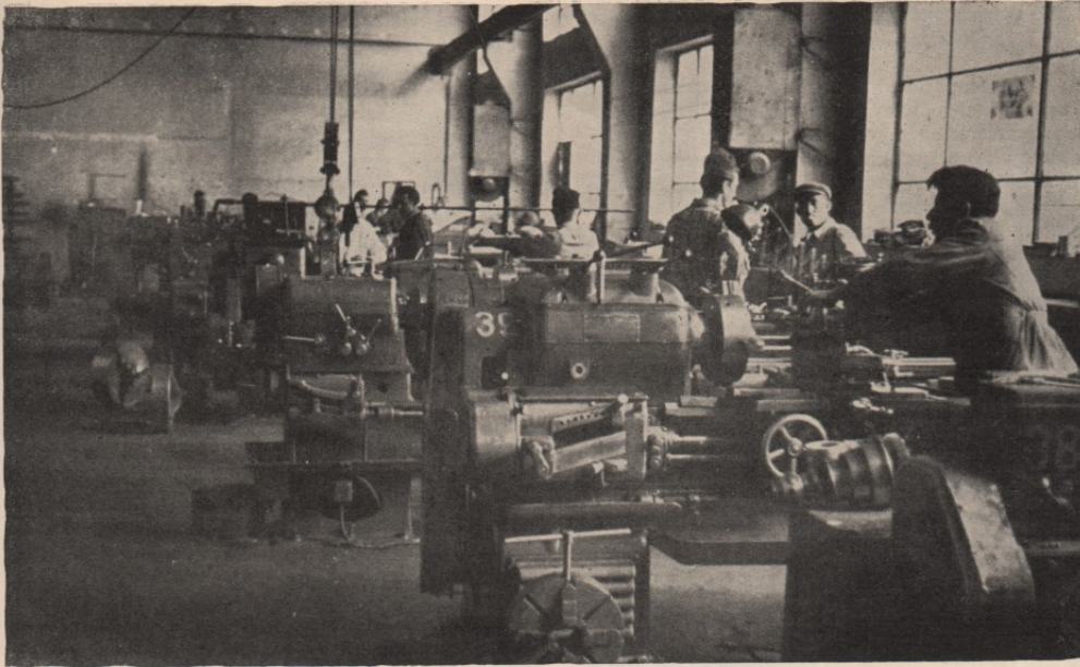
Стругарска радионица
